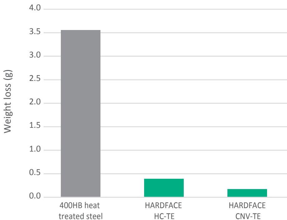
ASTM G65 Abrasion Test
